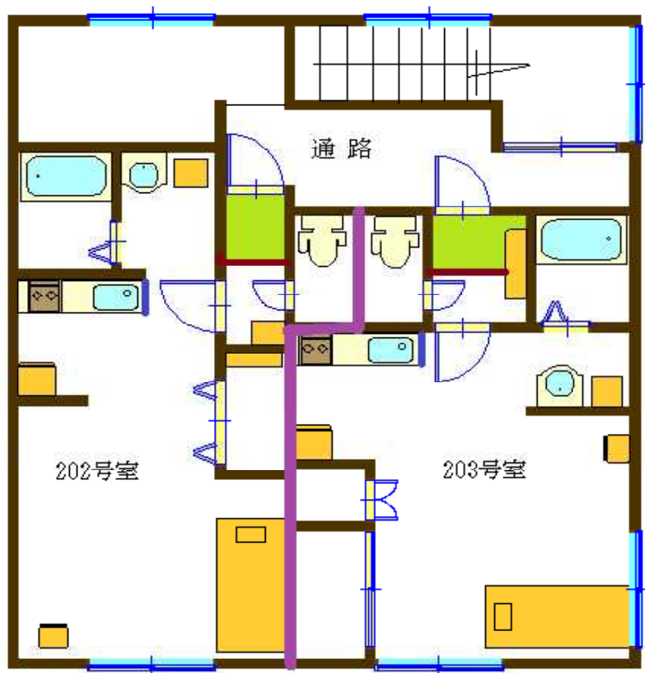
2階全体図
